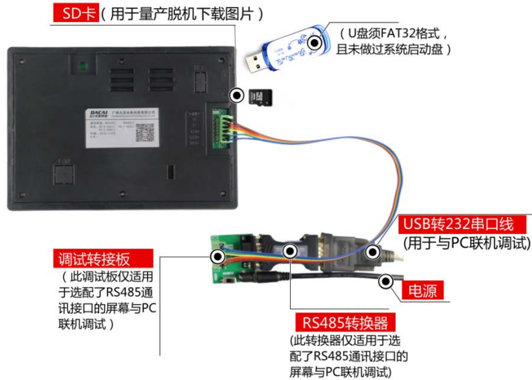
图 1-4 RS485 调试工具图
