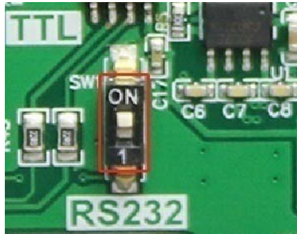
图 8-1 RS232/TTL 电平
